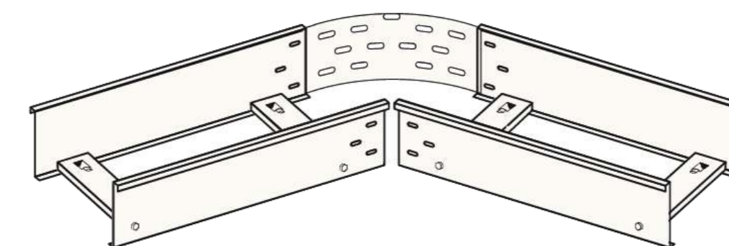
Curva Horizontal Ajustable (HA)
