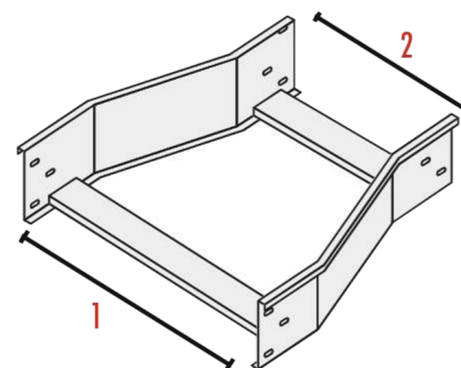
Reducción Simétrica (RS)
