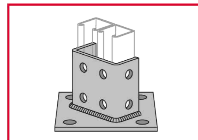
Base Poste para Canal Doble
